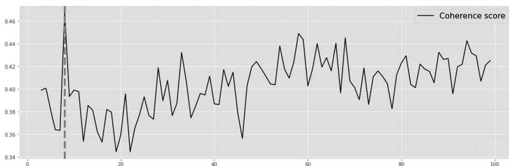
Рисунок 1 Степень когерентности LDA-модели в зависимости от количества тем
